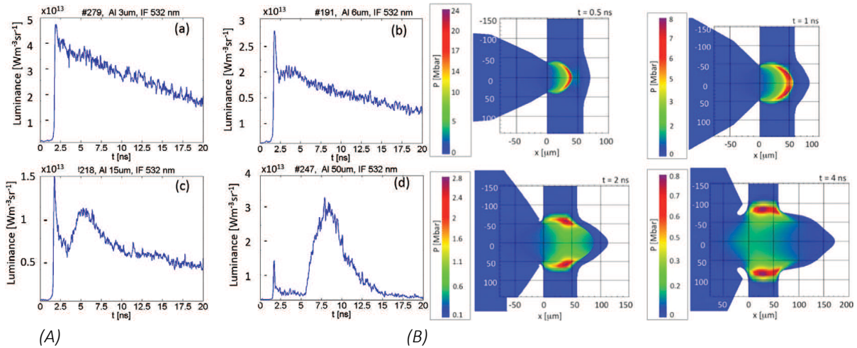
Rysunek 12: (A) Czasowy profil sygnału zmierzonego przy pomocy kamery smugowej dla tarczy aluminiowej o różnej grubości (a) 3 μm, (b) 6 μm, (c) 15 μm, (d) 50 μm pokazujący zachowanie ostrego piku i późniejszej emisji własnej w zależności od grubości tarczy. (B) Mapy ciśnienia 2D dla t = 0,5, 1, 2 i 4 ns dla tarczy aluminiowej o grubości 50 μm. Na początku oddziaływania lasera z tarczą powstaje fala uderzeniowa. Po około 2 ns, z powodu szybkiego rozszerzania się tarczy, struktura fali uderzeniowej zostaje utracona na osi symetrii ( r=0 ), a ciśnienie staje się bardziej jednorodne, ale jest utrzymywane poza osią oddziaływania lasera z próbką materiału.
